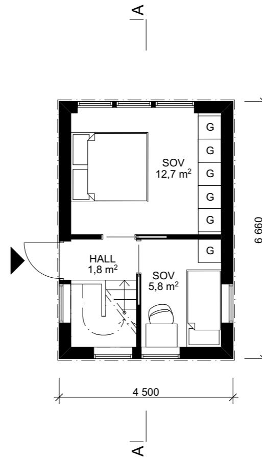
ÖVREPLAN SKALA 1:100
