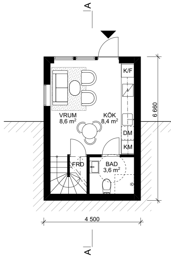
ENTRÉPLAN SKALA 1:100
