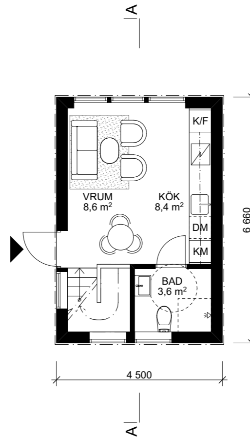
ENTRÉPLAN SKALA 1:100
