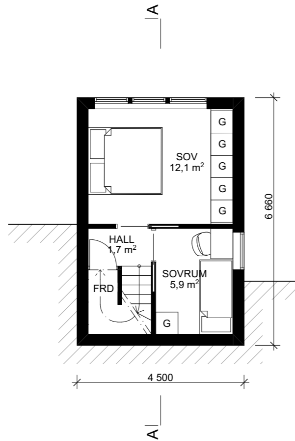
NEDREPLAN SKALA 1:100
